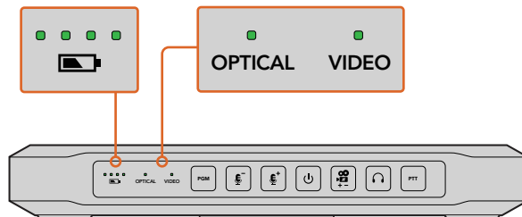
图为电池电量、光纤信号以及视频信号状态提示灯。
