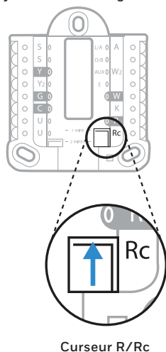
Curseur R/Rc
