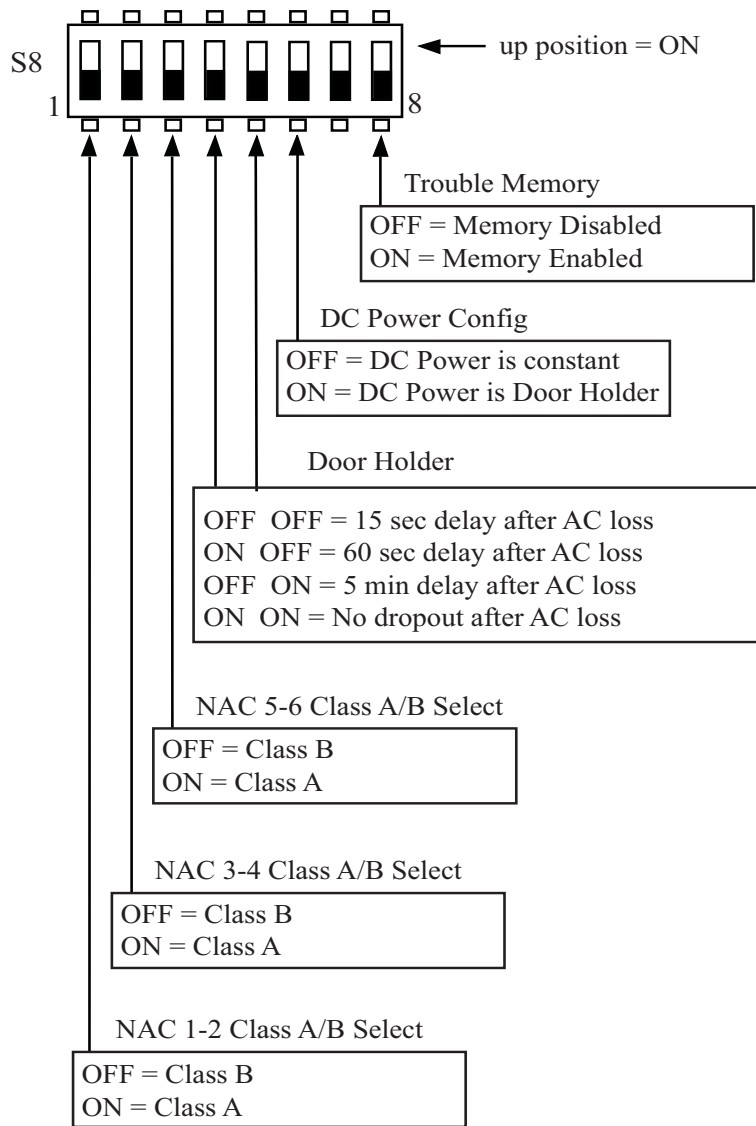
DWG# 3590-16
