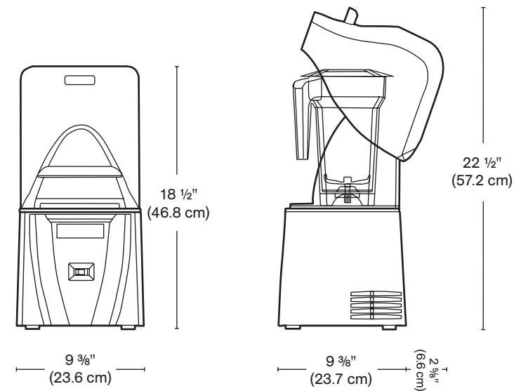
Figure 4. Connoisseur 825 Dimensions
