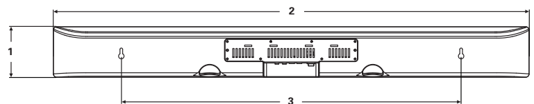
Barra montada en la pared
