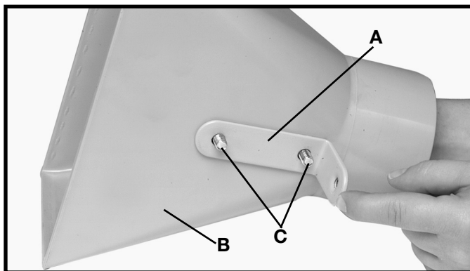
5. Sujete el anclaje del angular del soporte de la entrada al embudo de entrada introduciendo los dos pernos de carruaje de cabeza semiesférica de 5/16-18x5/8" (C) a través del embudo de entrada (B) y el anclaje del angular del soporte de la entrada (A), de la manera que se muestra en la Fig. 11.
