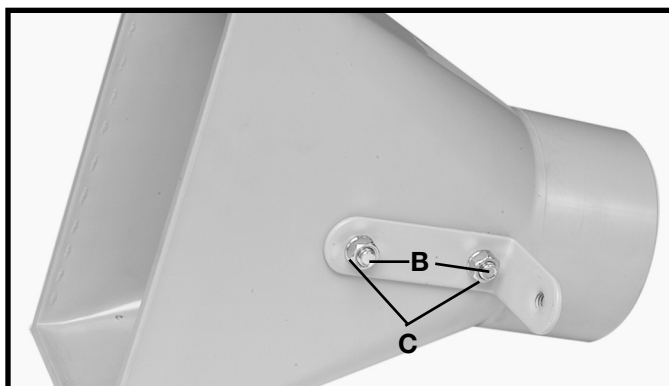
6. Enrosque una tuerca hexagonal reborde de 5/16" (C) Fig. 12 en el perno (B) y apriétela firmemente.
