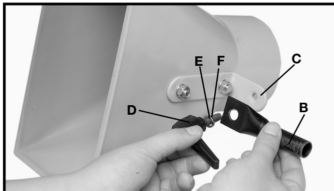
7. Sujete la ménsula del soporte superior (B), Fig. 13, al angular del soporte de la entrada (C) con la palanca de fijación ajustable (D). NOTA: COLOQUE UNA M8.4 ARANDELA PLANA (E) ARANDELA DE SEGURIDAD DE 5/16" (F), FIG. 13, EN EL TORNILLO DE LA PALANCA DE FIJACIÓN ANTES DE REALIZAR LA SUJECIÓN AL ANGULAR DEL SOPORTE DE LA ENTRADA.
