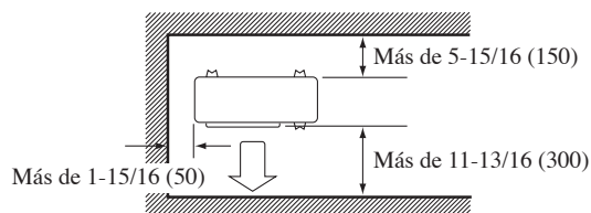
Vista superior
