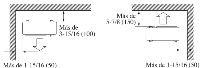
Vista superior
